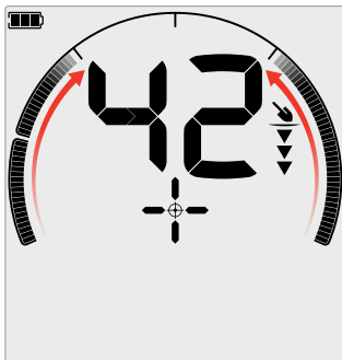
Isyarat sasaran yang lemah/luar pusat: Sedikit segmen beza layan Dihidupkan. Sasaran terletak lebih dekat dengan bahagian luar gegelung.
